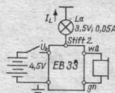
Bild 5: Hier ist der Bausatz zur Signalisierung vergessen-er Autoscheinwerfer eingesetzt
