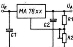
Bild 12: Einstellbare erhöhte Ausgangsspannung (u. l.)
