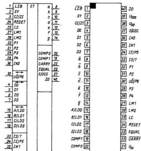
Bild 1: Schaltsymbol des U 125 D
