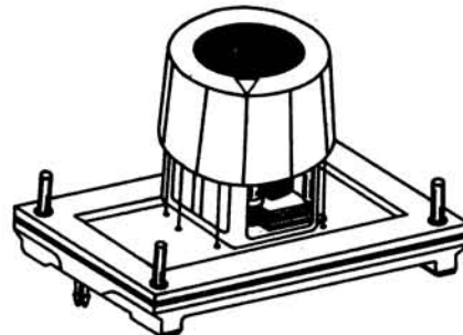
Bild 21: Anordnung des Drehkondensators auf dem Bauelementeträger
