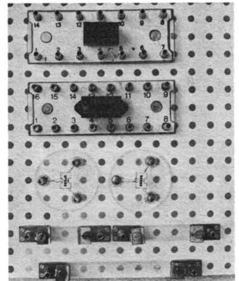
Bild 23: Universell einsetzbare Bauelementeträger für IS, Transistoren und diskrete Bauelemente öffnen das System für Erweiterungen
