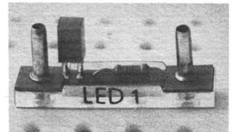
Bild 18: Als Anzeigebau-elemente kommen überwiegend LED zum Einsatz, die paarig antiparallel geschaltet mit dem erforderlichen Vorwiderstand auf dem Bauelementeträger angeordnet sind
