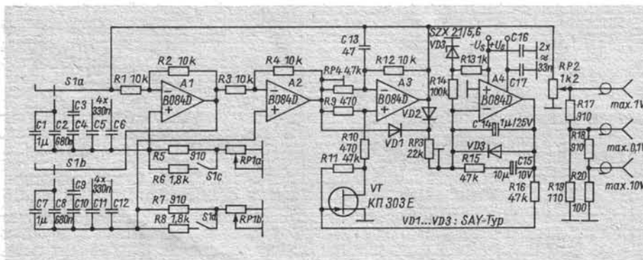
Bild 1: Hochwertiger Sinusgenerator. Die Kapazitäts-Beschaltung am Stufenschalter S1 ist ein Beispiel; mit C5, 6, 11, 12 verfährt man analog.
