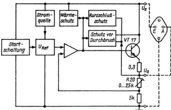
Bild 10: Grundschiung mit MA 78xx (o. l.)
