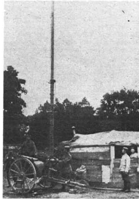
Eine „Feldtelefunkenstation“ aus der Zeit des 1. Weltkrieges Repro: K. Theurich
