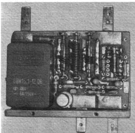
Bild 10: Ansicht eines vollständig bestückten Blinkgebers
