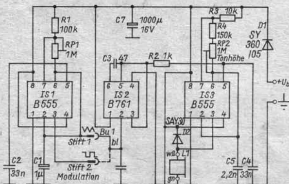
Bild 3: Auch als Türklingel ist der Generator einsetzbar
